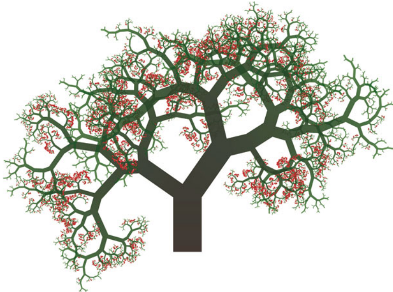
Verallgemeinerter Baum des Pythagoras (s.S. 95)
