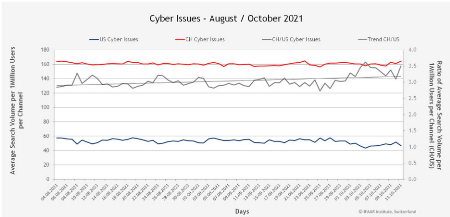
Abb. 6 Suchvolumen aller Cyberthemen (Risiken und Chancen) pro 1 Mio. Nutzer*innen
