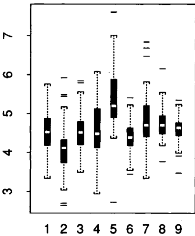
Fig 3. «Boxplots» des 9 classes agronomiques pour des variables observées en différents lieux (BL : Bourg-Lastic; LP : Le Pin au Haras).
