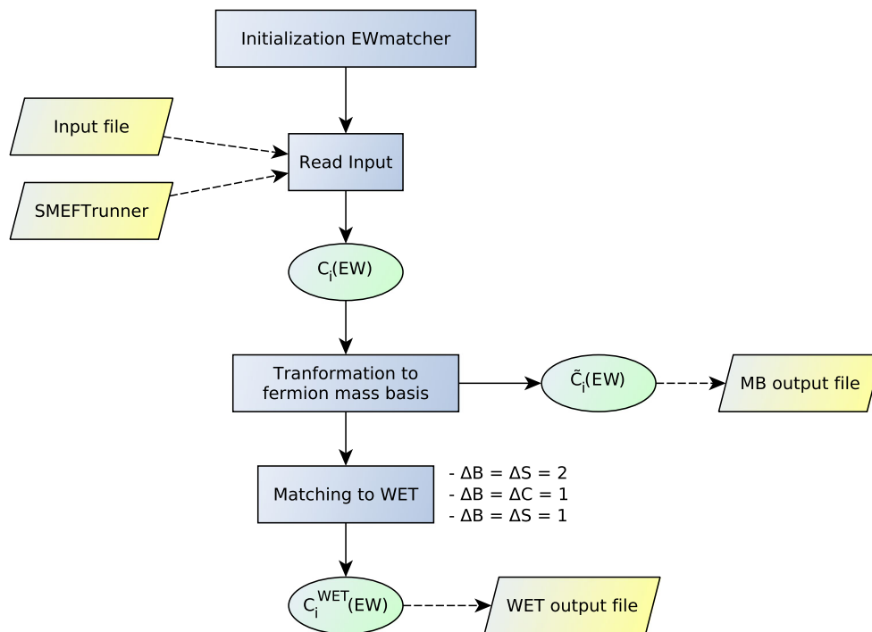
Fig. 4 EWmatcher module flowchart
