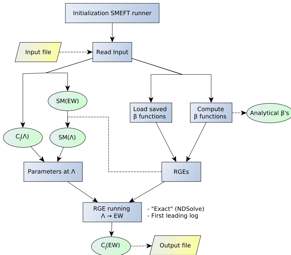
Fig. 3 SMEFTrunner module flowchart
