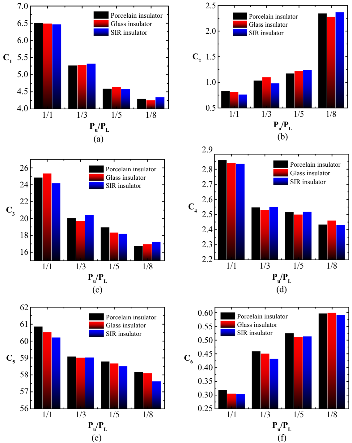
Figure 13. LC indicators versus P_u/P_L for tested insulators under SDD=0.2 \text{ mg/cm}^2 , NSDD=0.35 \text{ mg/cm}^2 and Wt=9 \text{ l/h} : (a) C_1 ; (b) C_2 ; (c) C_3 ; (d) C_4 ; (e) C_5 ; (f) C_6 .
