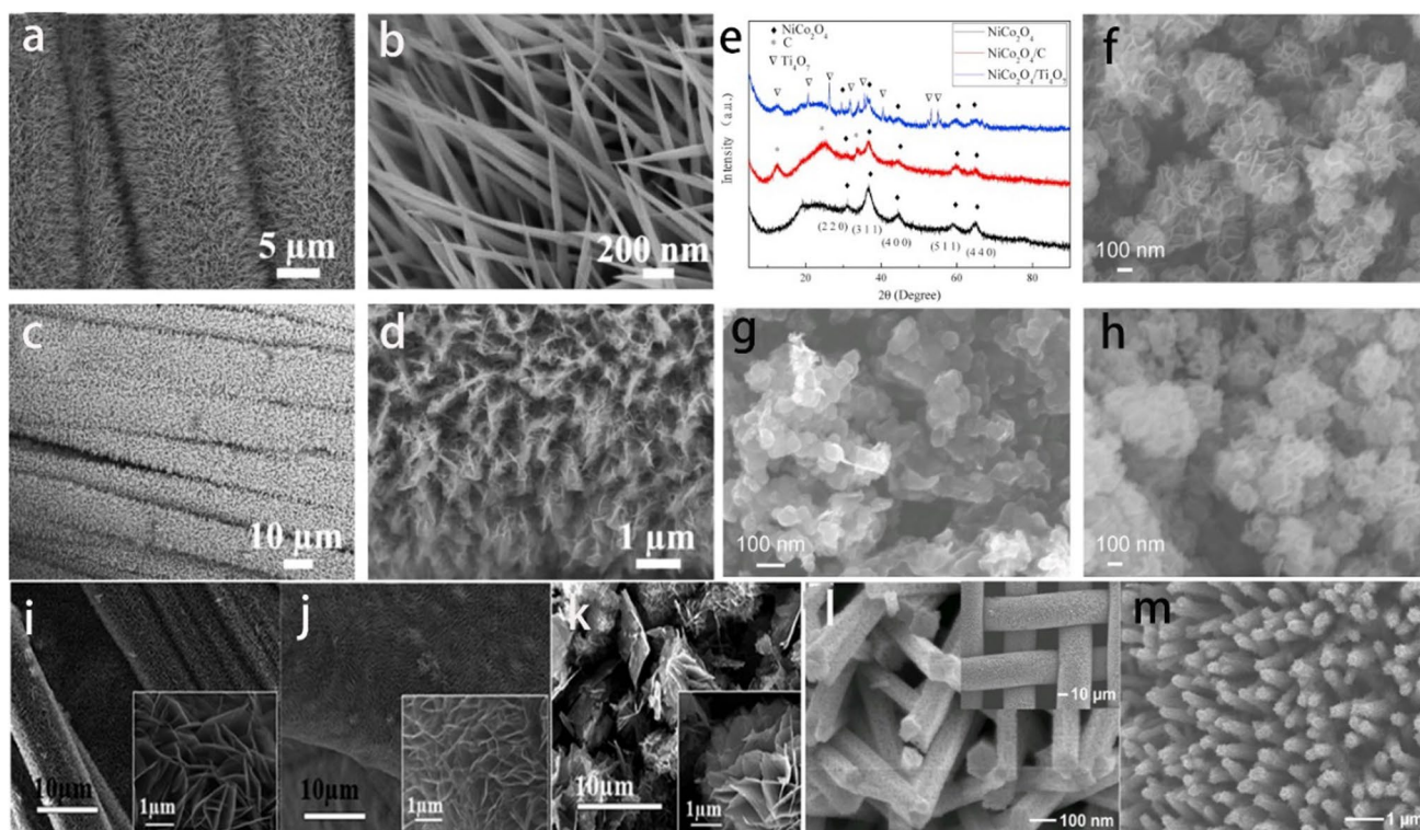
Fig. 6 a–d SEM images of NiCo 2 O 4 nanowire arrays [67]. e–h XRD patterns and SEM images of NiCo 2 O 4 , NiCo 2 O 4 /C and NiCo 2 O 4 /Ti 4 O 7 [66]. i–k SEM images of NiCo 2 O 4 /CP, NiCo 2 O 4 /NF and NiCo 2 O 4 nanosheets [70]. l–m SEM and TEM images of NiCo 2 O 4 /SSL [71]
