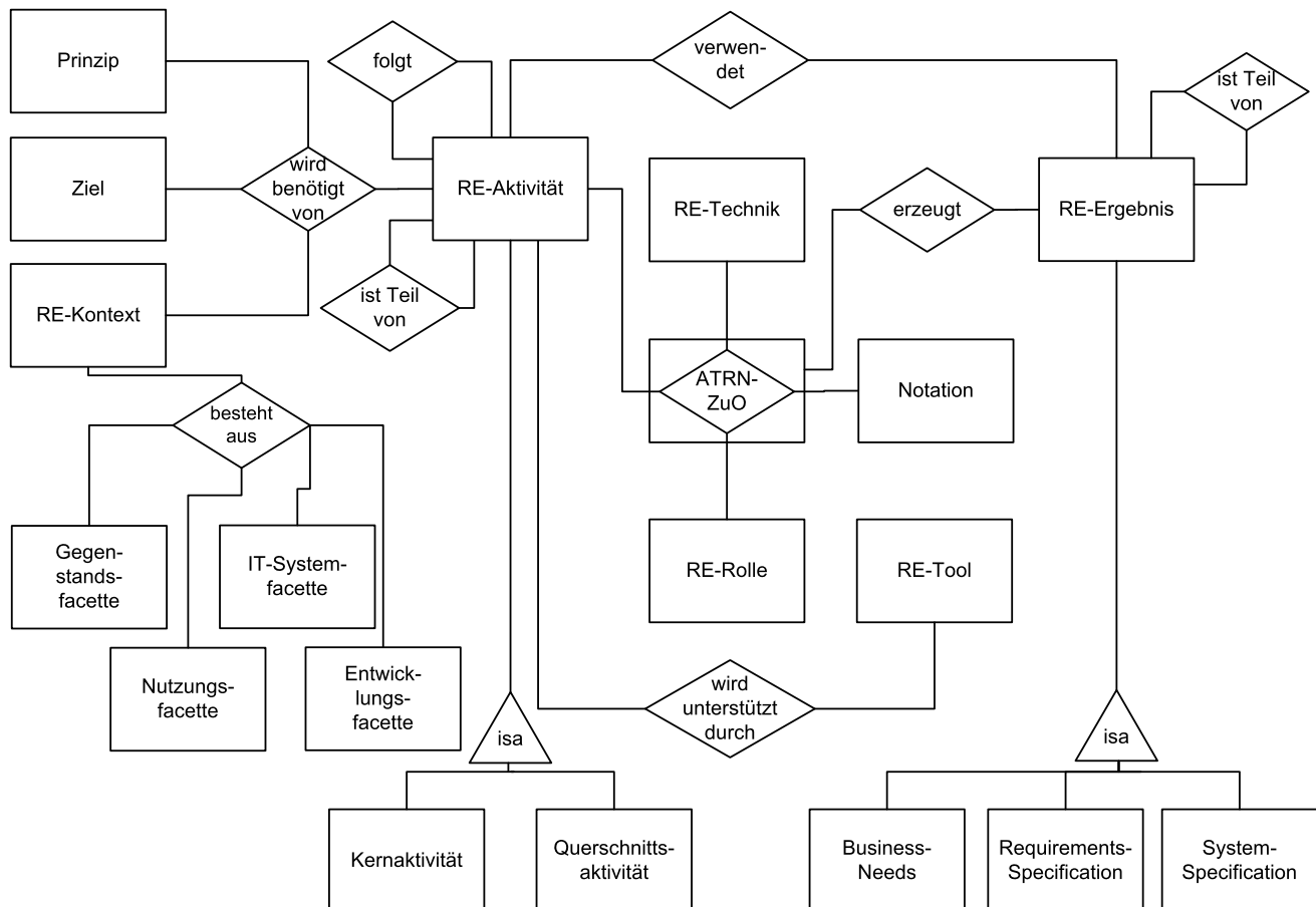
Abb. 2 Ordnungsrahmen zur Strukturierung empirischer Forschung im RE
