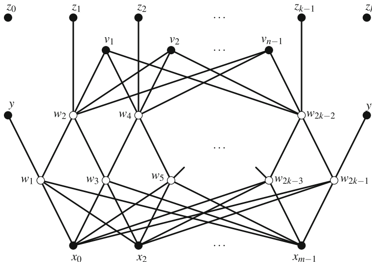
Fig. 4 Poset Q
