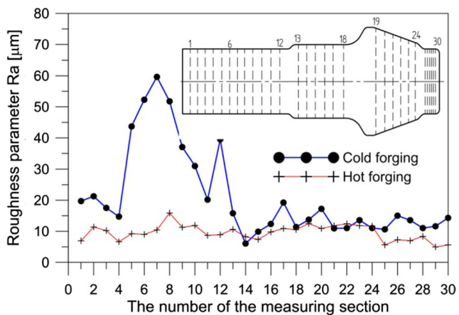
Fig. 14 Changes to the roughness parameter Ra
