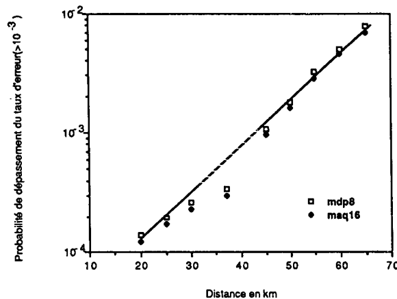
FIG. 1. — Variation théorique de la qualité d'une liaison témoin avec sa longueur (Marcheville-Viabon). Theoretical variation of the test link quality (Marcheville-Viabon) with distance.
