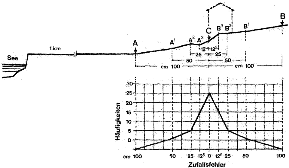
Abb. 5. Schematisches Beispiel der Verteilung zufälliger Fehler: das Gesetz von Gauss.
