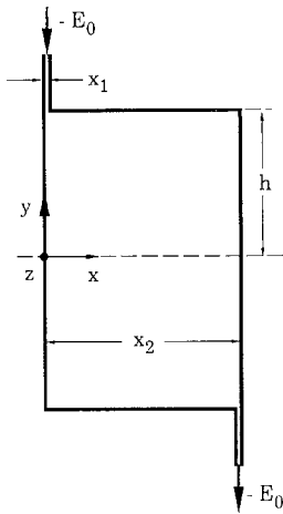
Bild 4. Diagonal eingespeister Flächenleiter
