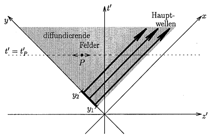
Bild 3. Ausbreitung der unterschiedlichen wellenterme der rechts laufenden Basiswelle
