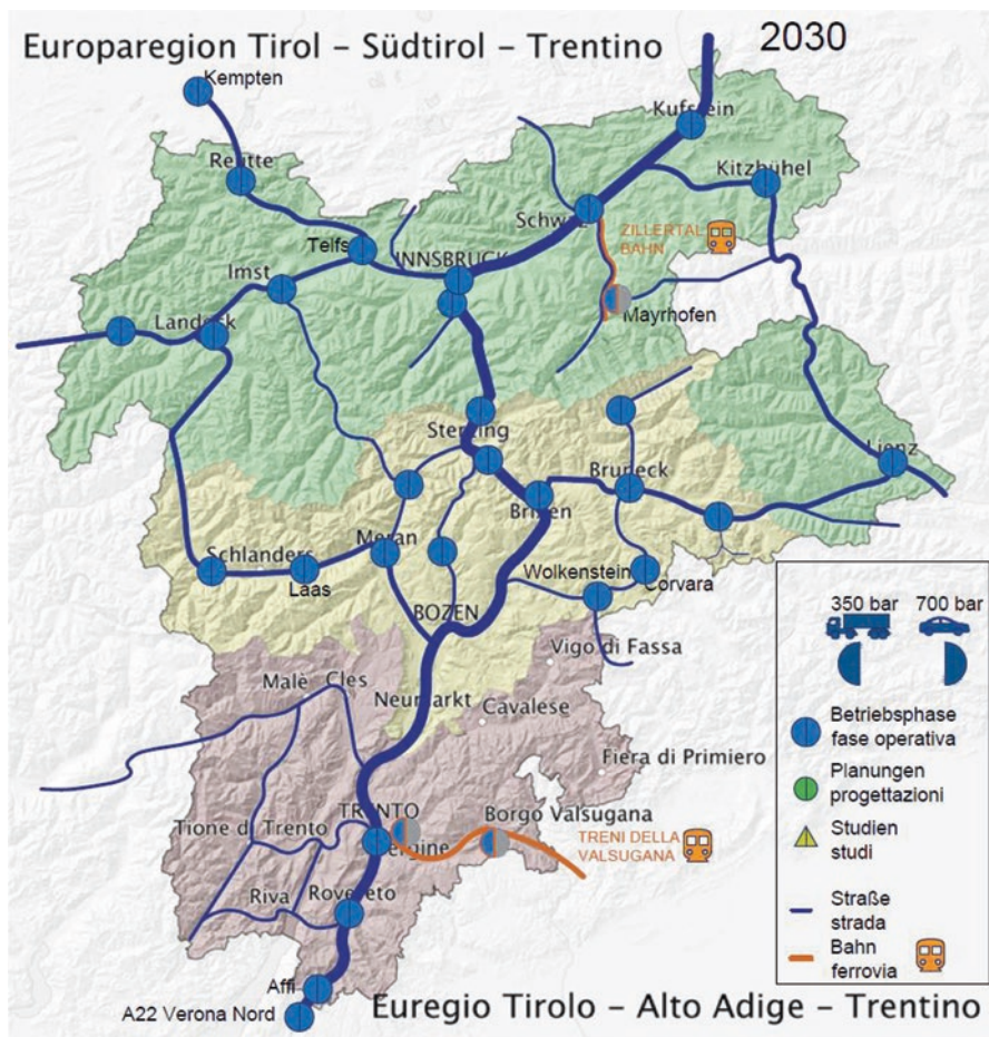
Abb. 4 Umsetzung der H2-Strategie in der Euregio Tirol-Südtirol-Trentino; Stand 2030
