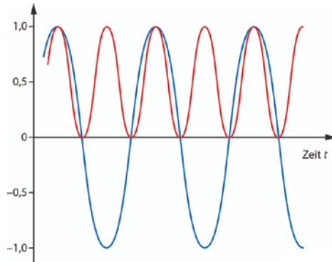
■ Abb. 1.13 Sinus (auch ins negative gehender Graph) und Sinus quadrat (Graph nur im Positiven)
