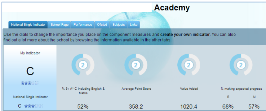
Fig. 5. NSI tab
