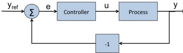
Fig. 1. Feedback loop
