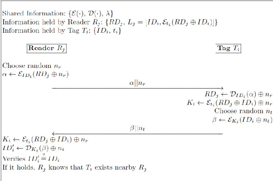
Fig. 1. Chun et al.'s RFID tag search protocol
