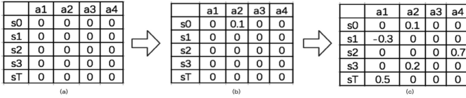
Fig. 2. Q(s, a) function
