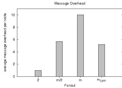
Fig. 6. Message Overhead
