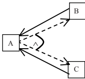
Fig. 12. Xor-Split.
