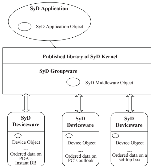
Fig. 1. SyD Framework.
